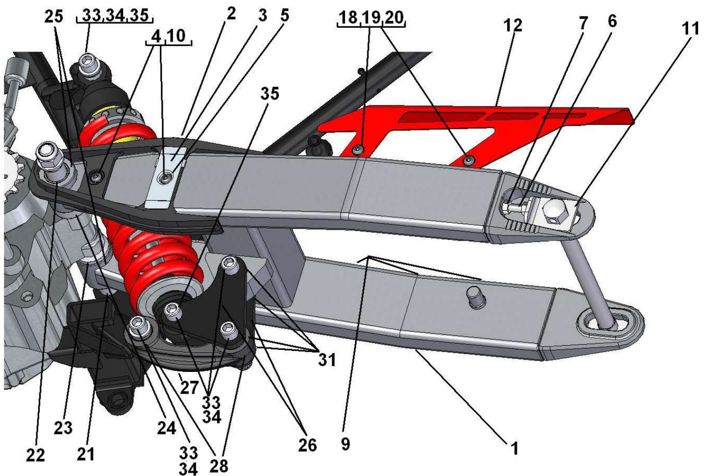
Obrázek č. 1: Pozice jednotlivých dílů na vidlici JAWA
